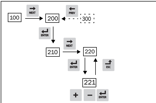
Figur 1 Exempel på menynavigering för att ange motorspänning
